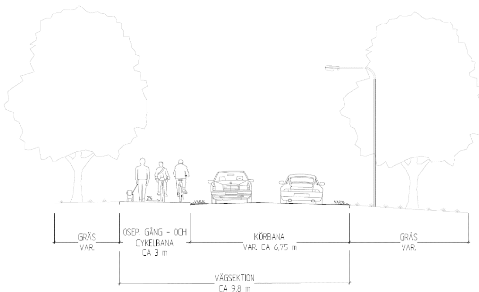
Figur 18. Typsektion för Siriusgatan, sektion A, vy österut.
