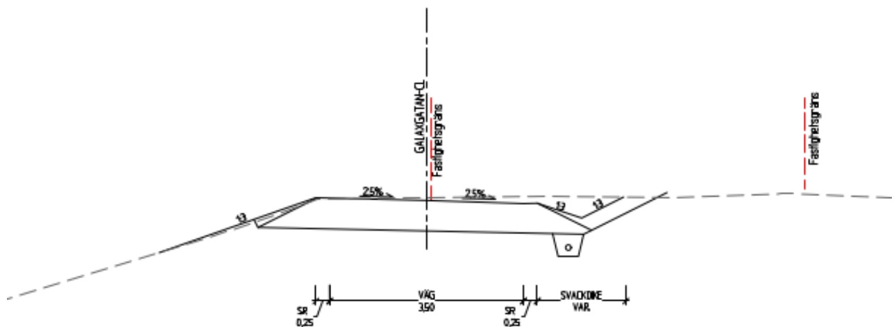
Figur 23. Typsektion för västra delen av Galaxgatan, sektion F, vy österut.
