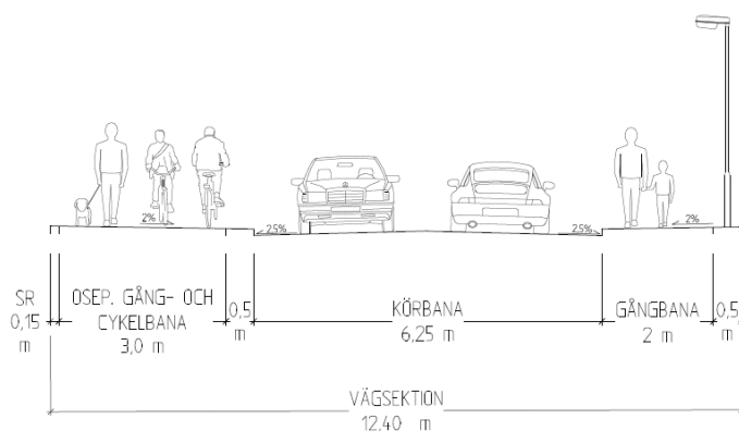
Figur 19. Typsektion för Siriusgatan, sektion B, vy österut/norrut.
