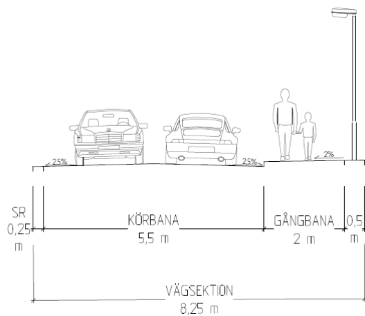
Figur 22. Typsektion för norra delen av ny lokalgata, sektion E, vy norrut.
