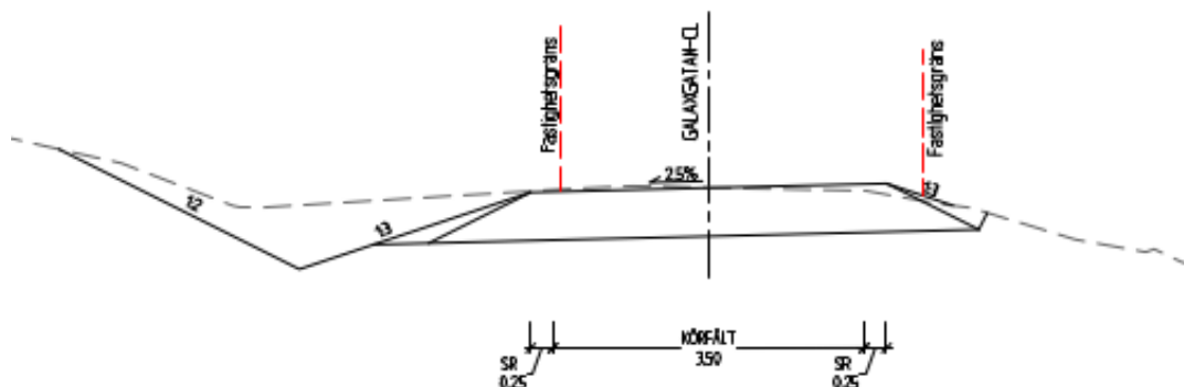
Figur 25. Typsektion för södra delen av Galaxgatan, sektion H, vy söderut.
