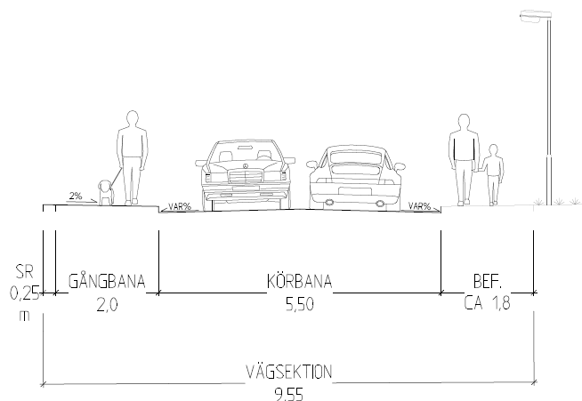
Figur 20. Typsektion för Siriusgatan, sektion C, vy norrut.
