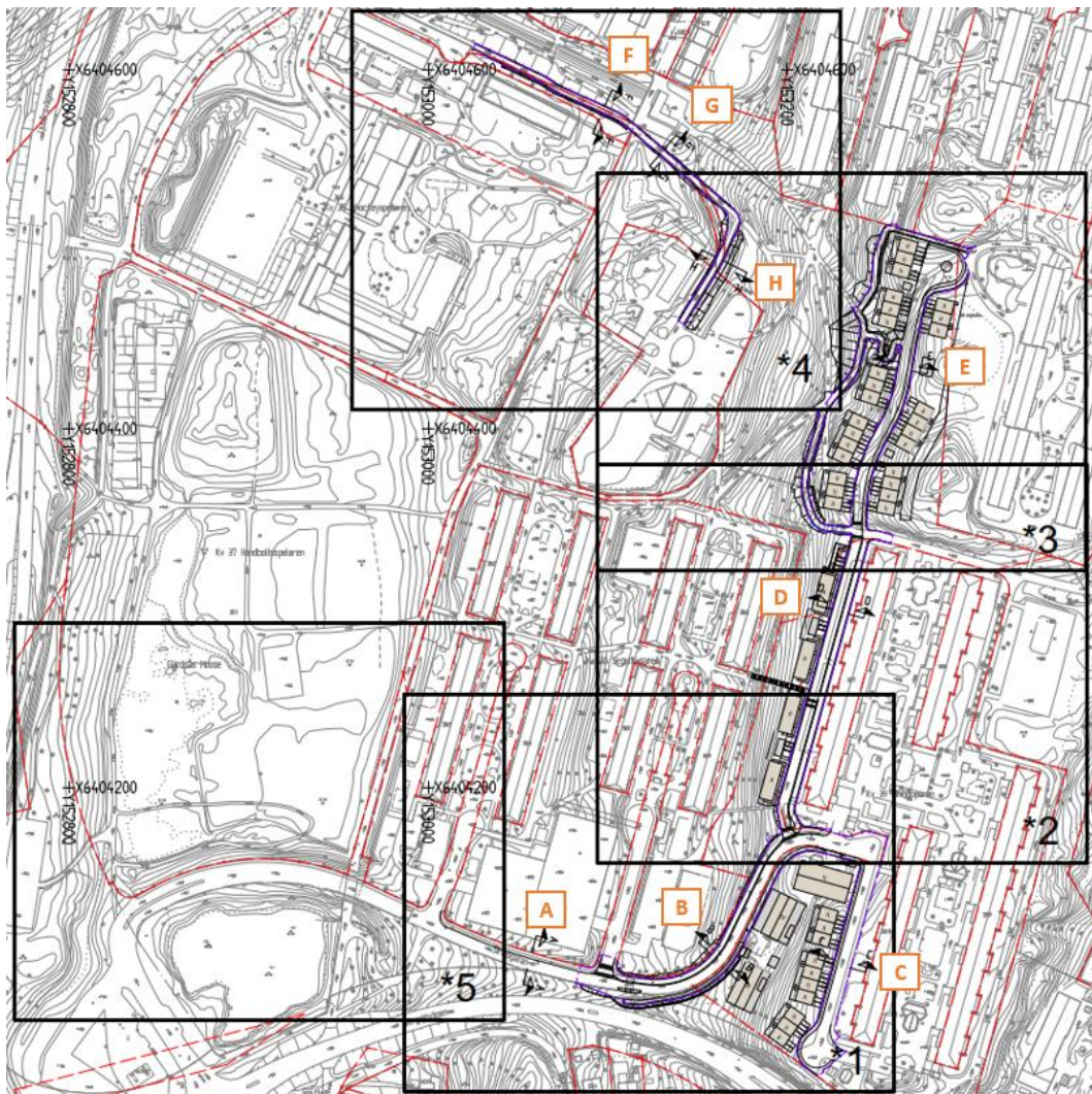
Figur 17. Översiktsritning inkl. arkitektförslag daterat 2022-04-29 med markering för de olika typsektionerna i trafikförslaget.
