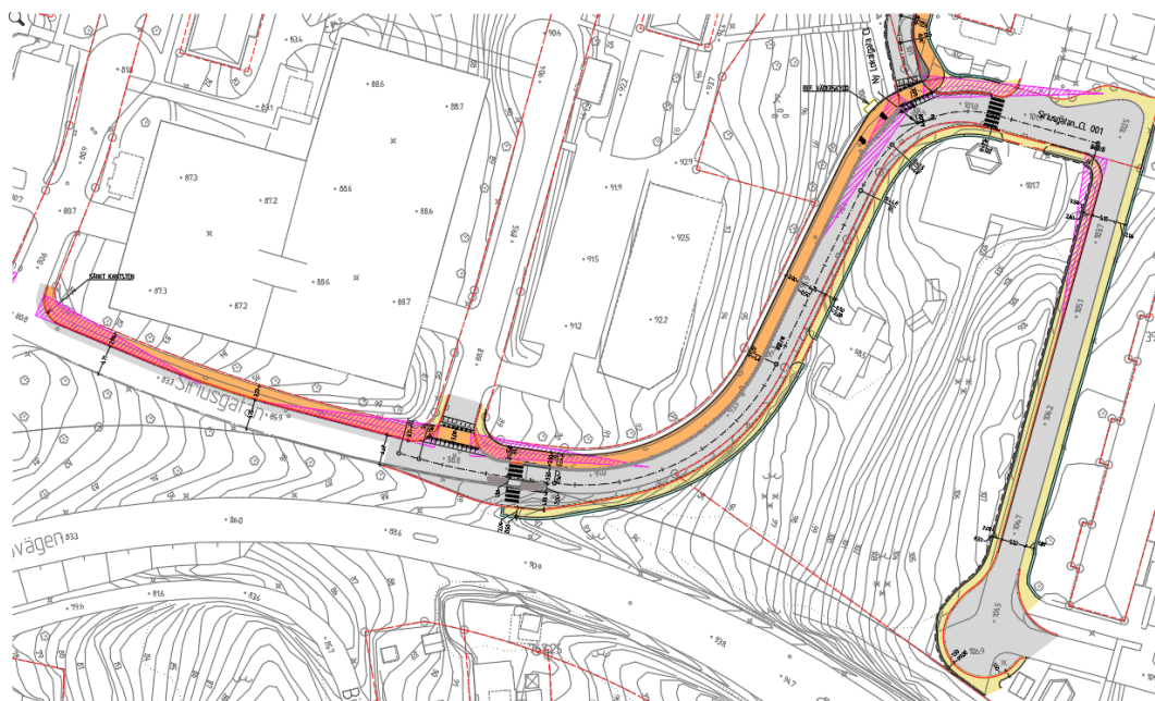
Figur 28. Sikttrianglar för hastighet 50 km/tim på primärgata vid ny föreslagen utformning.
