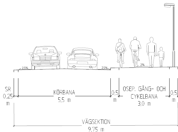
Figur 21. Typsektion för södra delen av ny lokalgata, sektion D, vy norrut.
